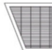
MOD.13 TRAPEZIO RETTANGOLO
